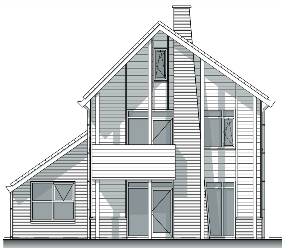
voorgevel
