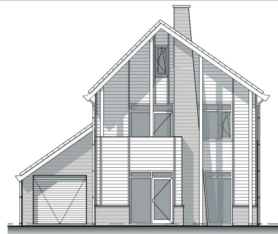
voorgevel
