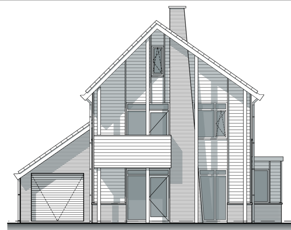
voorgevel
