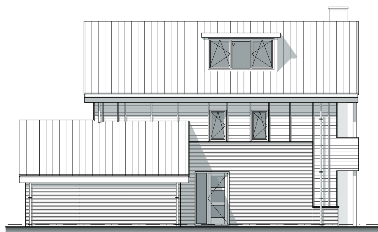
linkergevel
